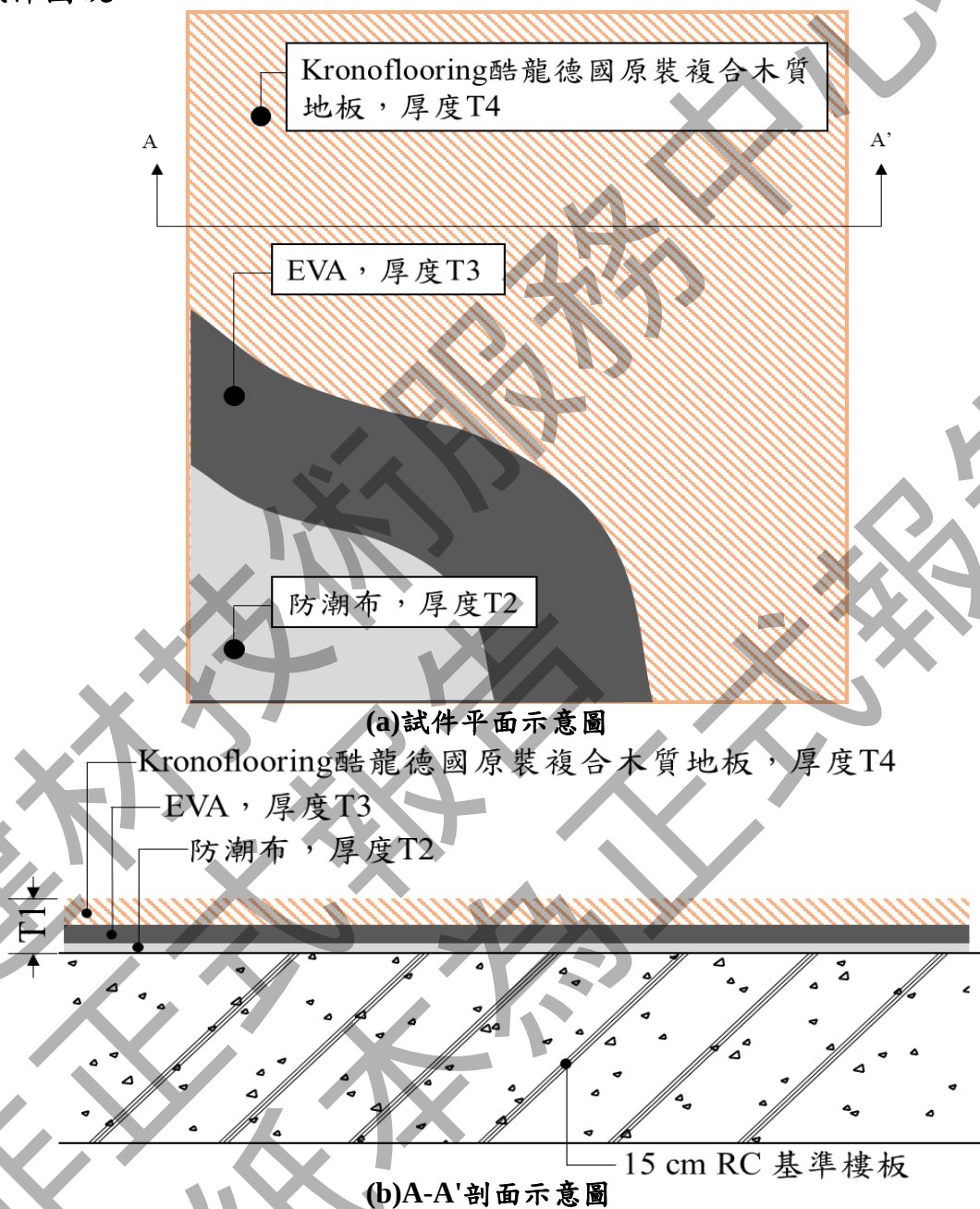
圖5.1 試件平面、剖面示意圖
