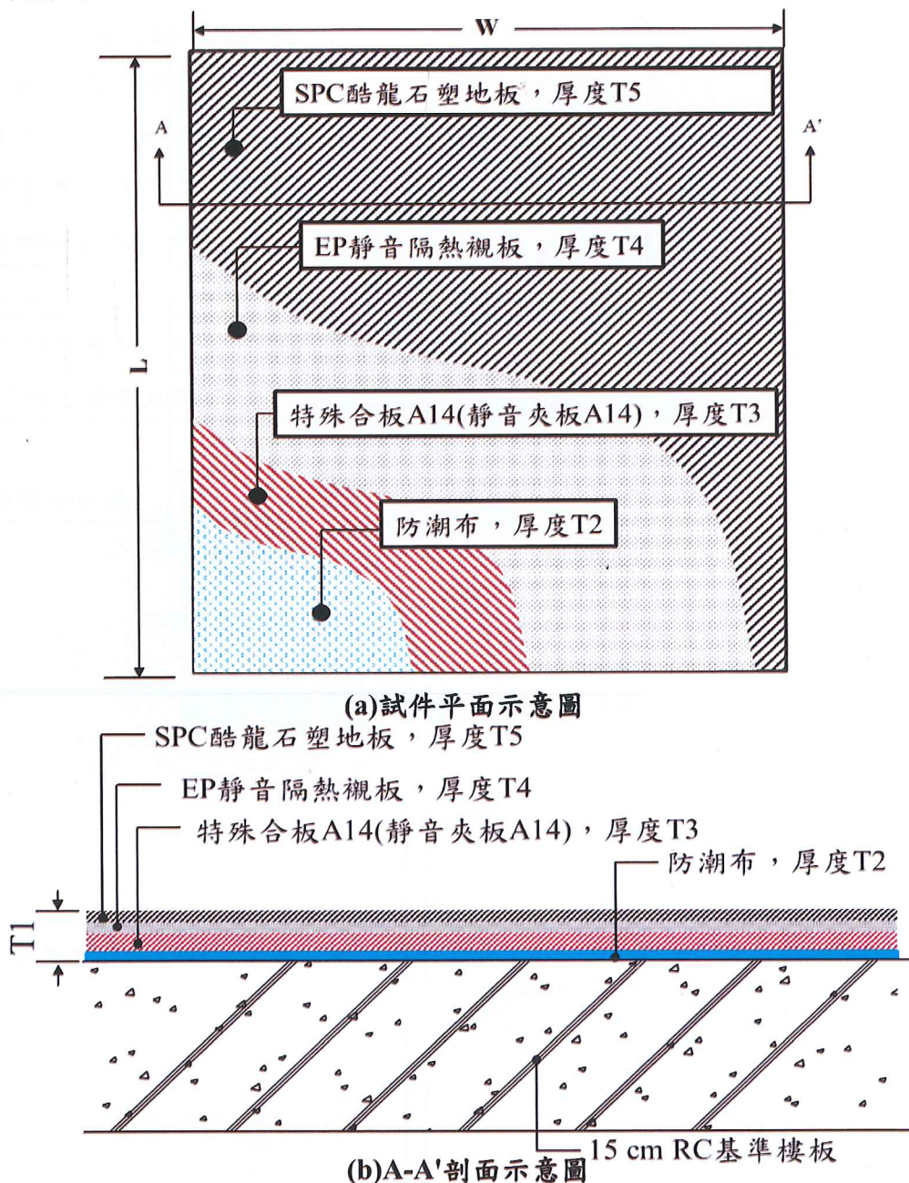
圖5.1 試件平面、剖面示意圖
